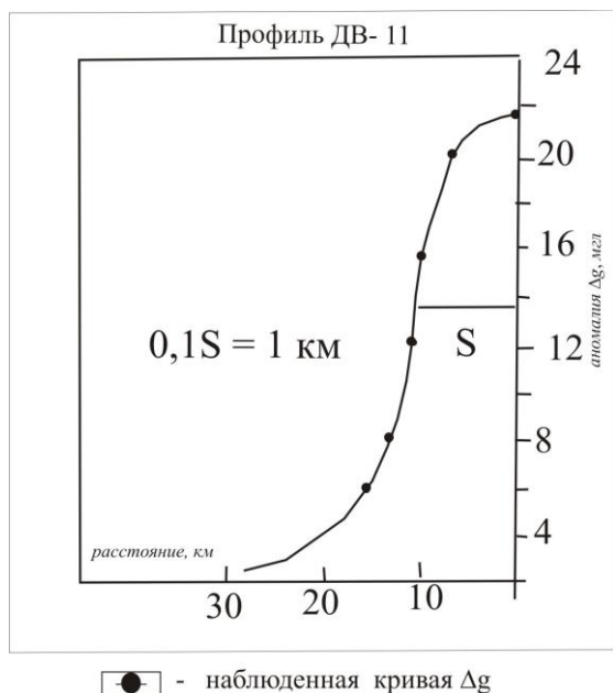
Рисунок 2 – График зависимости аномалии силы тяжести от расстояния вдоль профиля ДВ-11
