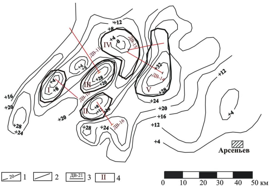
Рисунок 1 – Фрагмент карты аномалий силы тяжести в редукции Буге (Приморский край)
